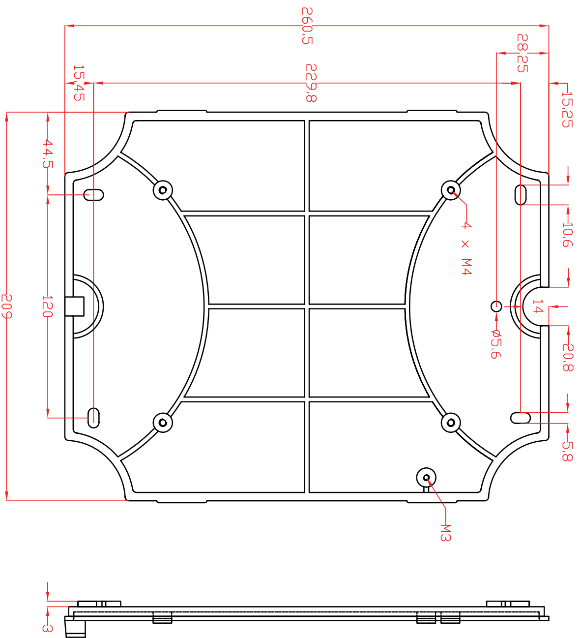
Gehäuseboden Kunststoffgehäuse ZPA
